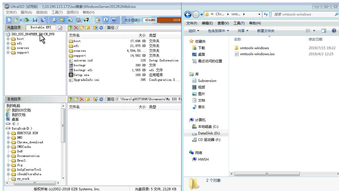
图 14 添加“vmtools-windows”文件夹至 ISO 镜像文件中
