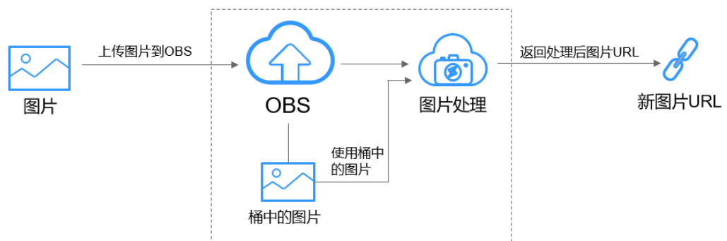
图1-1 图片处理架构
